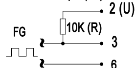
Tach output (FG)
