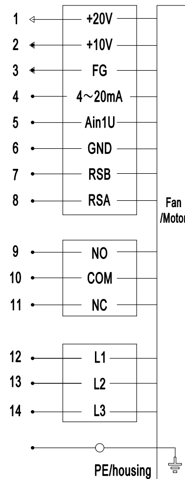
连接器 Connection
